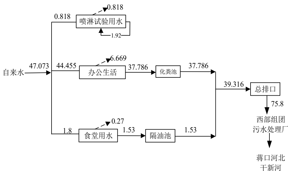
图 2-1 本项目水平衡图 (单位: m³/d)
