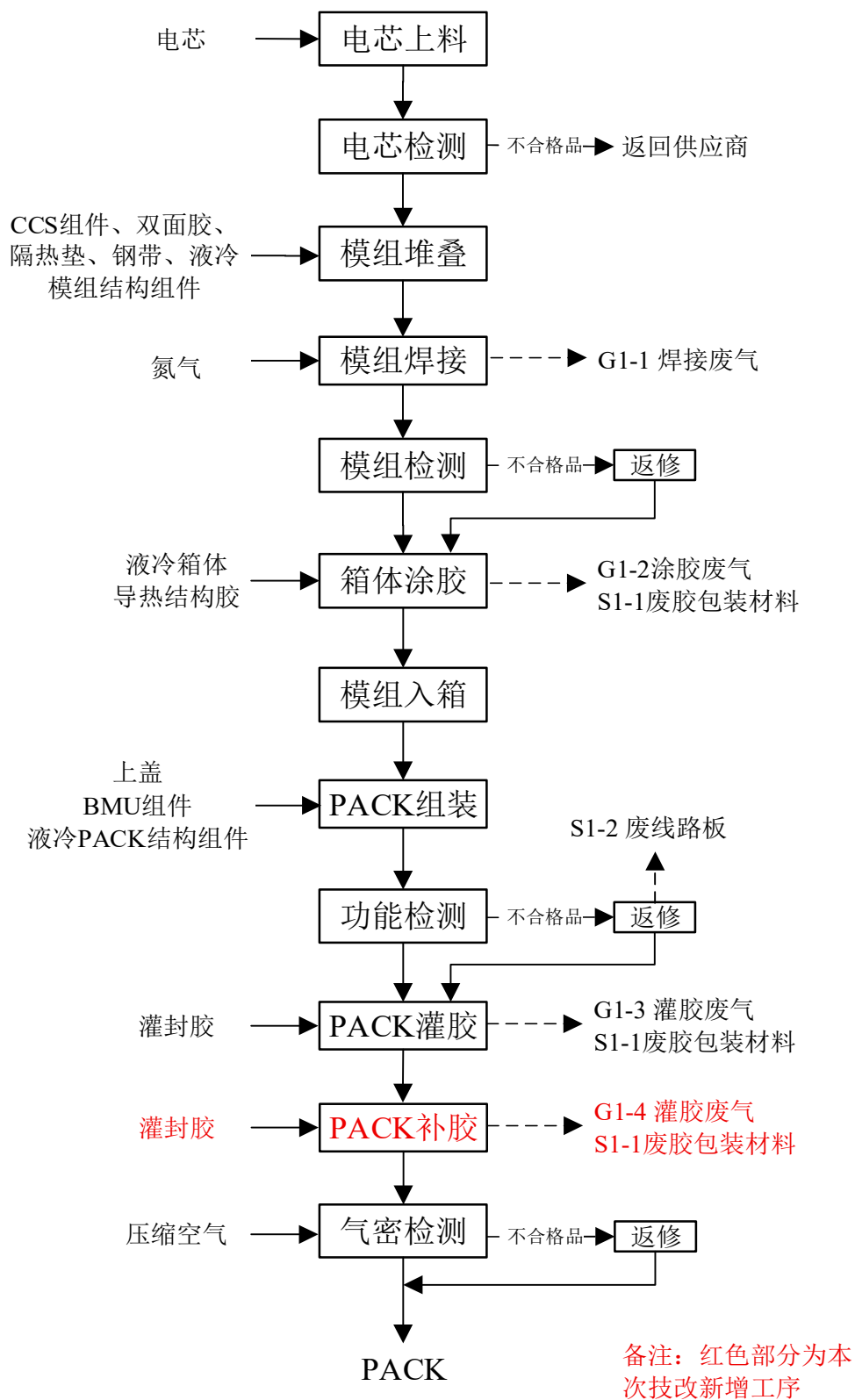
图 2-4 PACK 生产工艺流程及产污节点图
